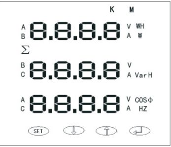
面板显示图
